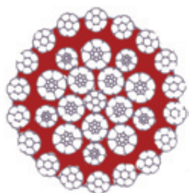
Câblage croisé
